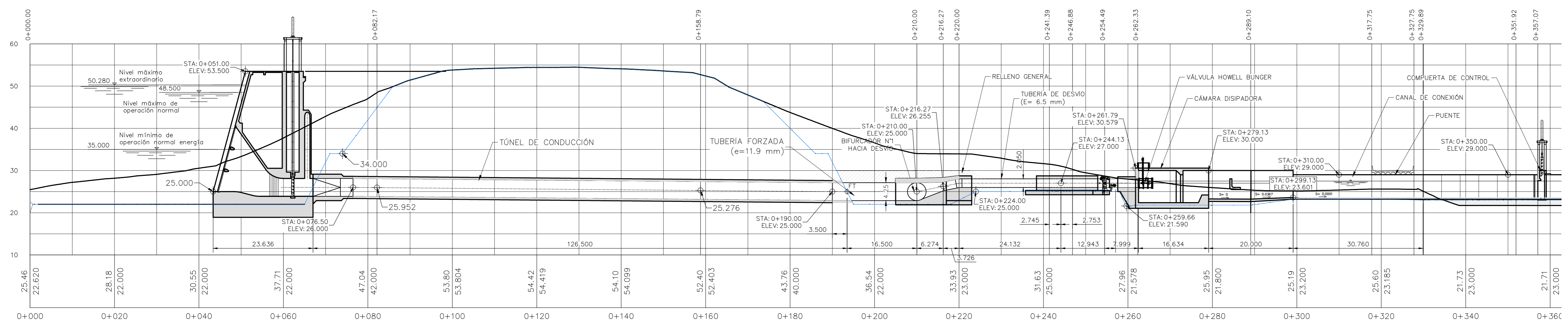
PERFIL LONGITUDINAL DE LA TOMA DE AGUAS, CONDUCCION Y CASA DE MAQUINAS
