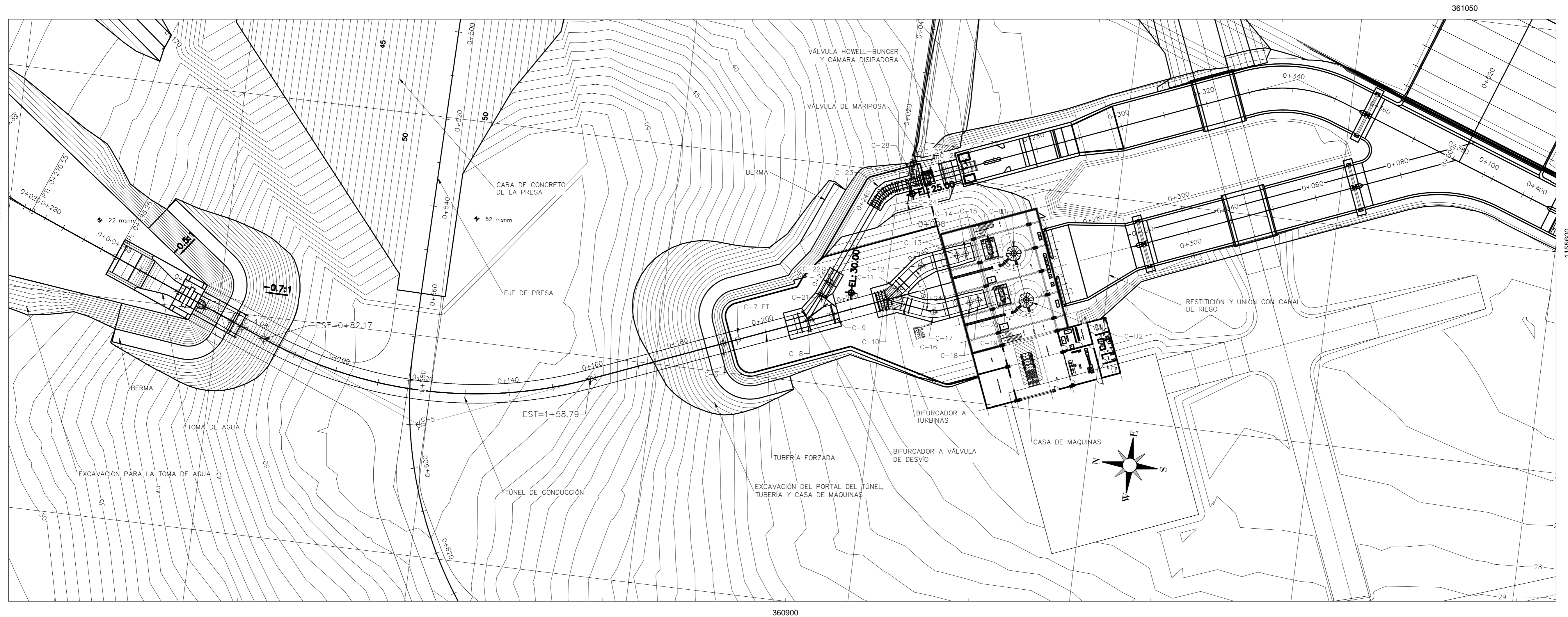
VISTA EN PLANTA DE LA TOMA DE AGUAS, CONDUCCION, DESVIO, CANAL DE RESTITUCION Y CASA DE MAQUINAS
